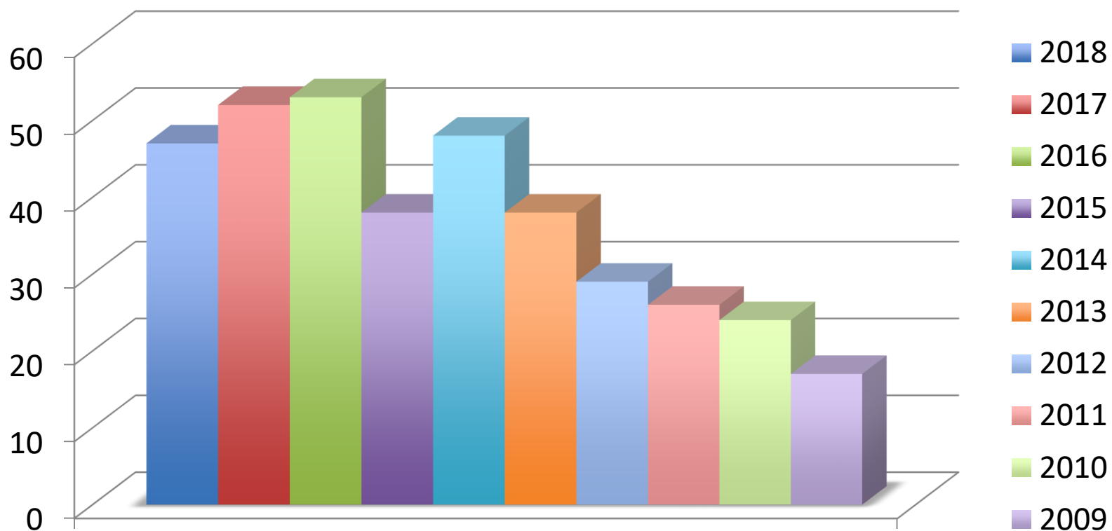
Artículos VIH-EPOC
